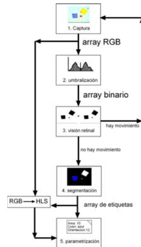
Figura 3. Flujo del proceso de reconocimiento visual.
